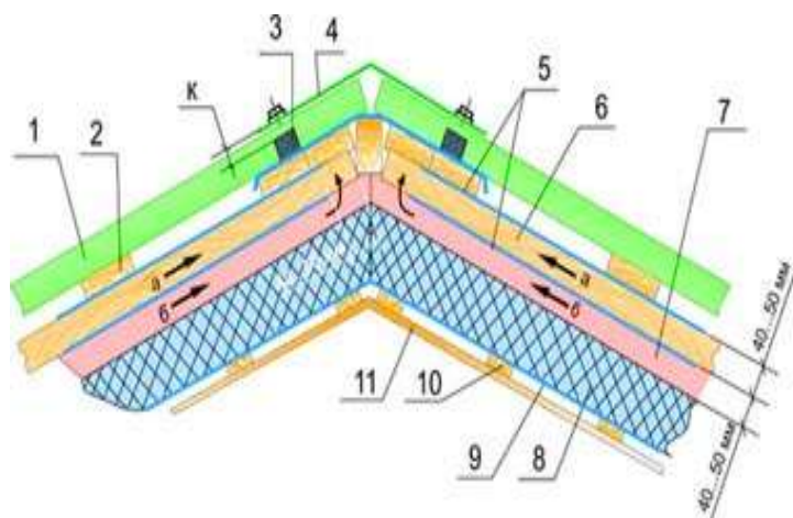
Рис.5 Утепление кровли
